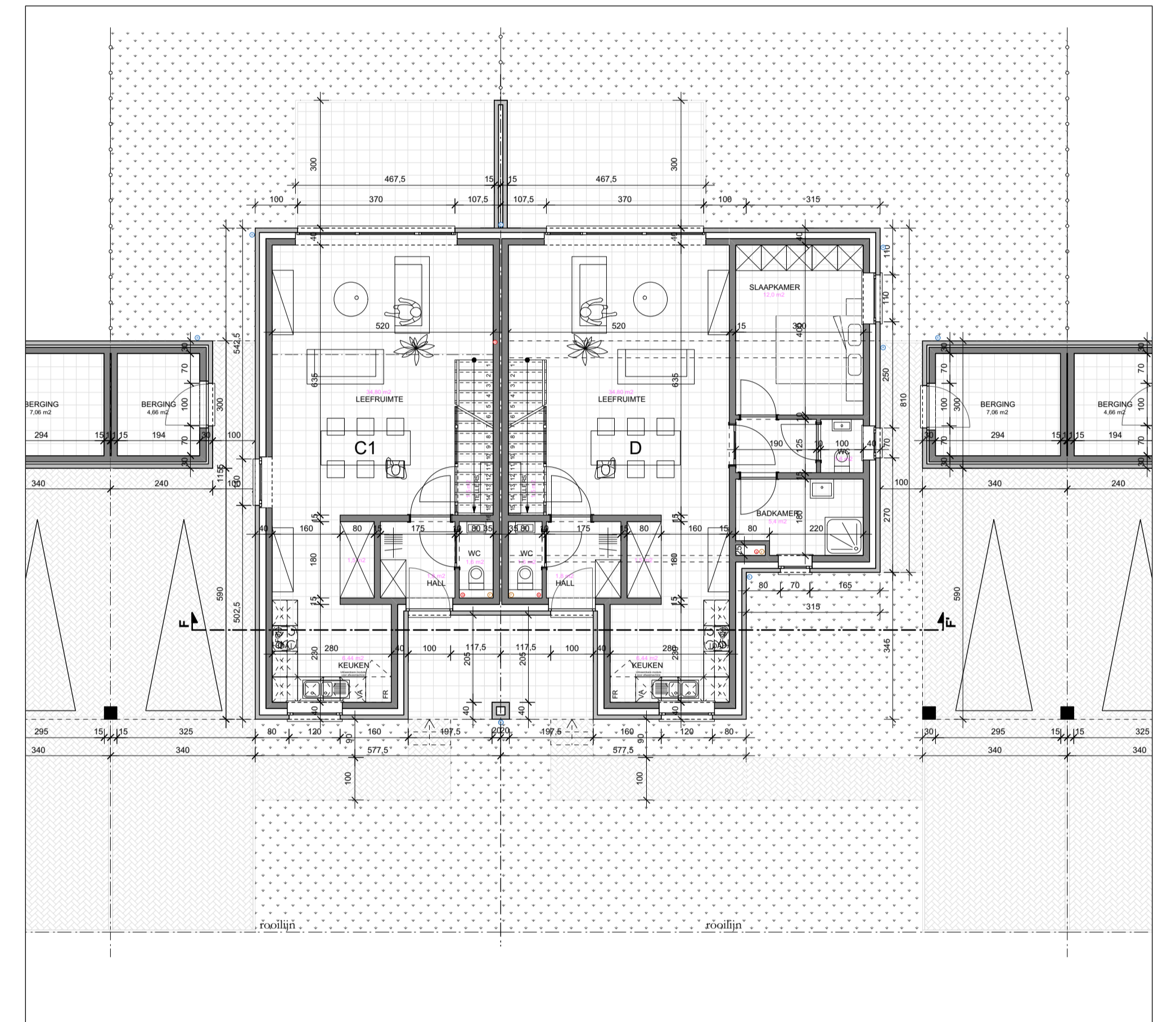
Typeschakeling CD + carports - GELIJKVLOERS
