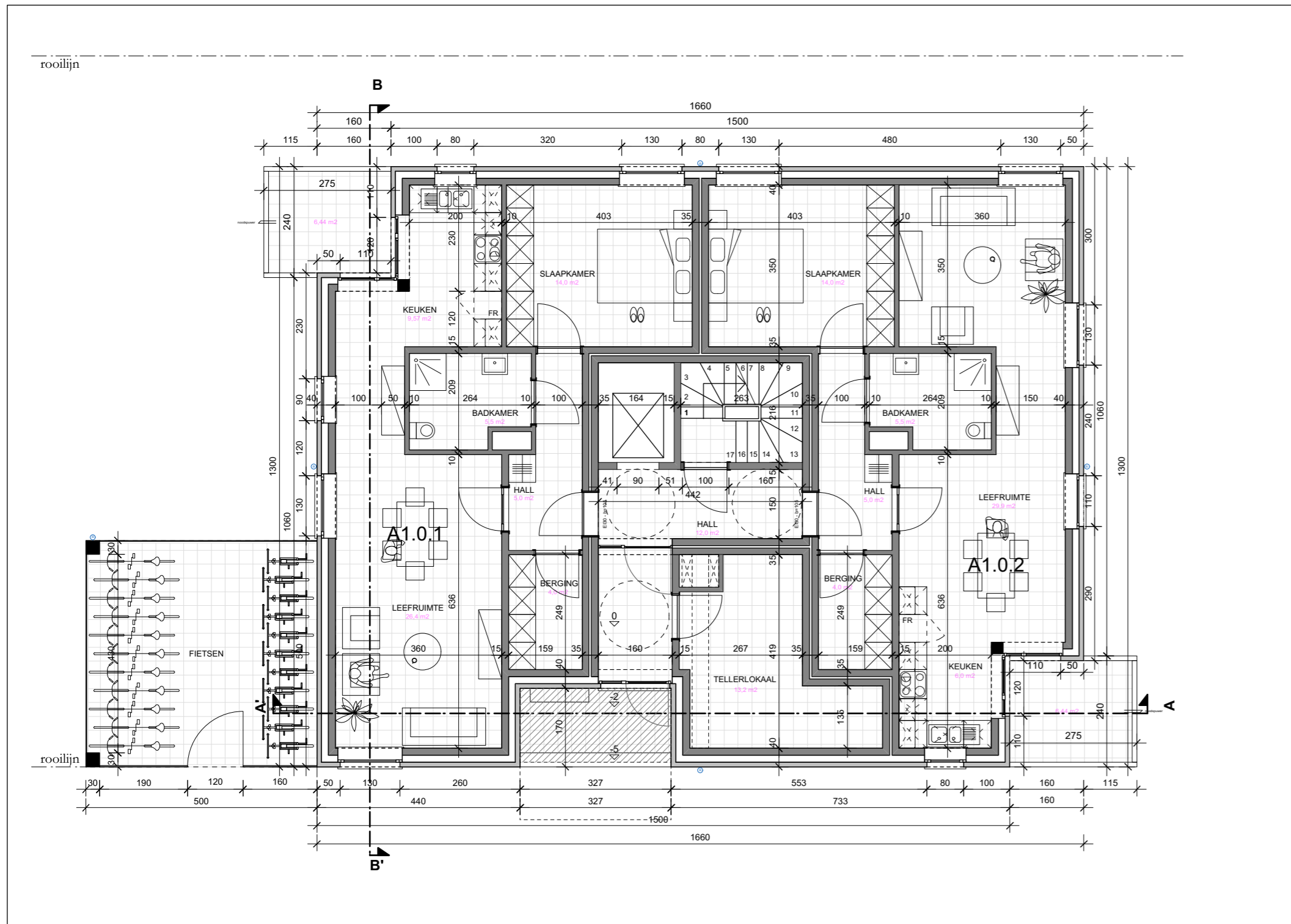
Appartementen Type A1 - GELIJKVLOERS
