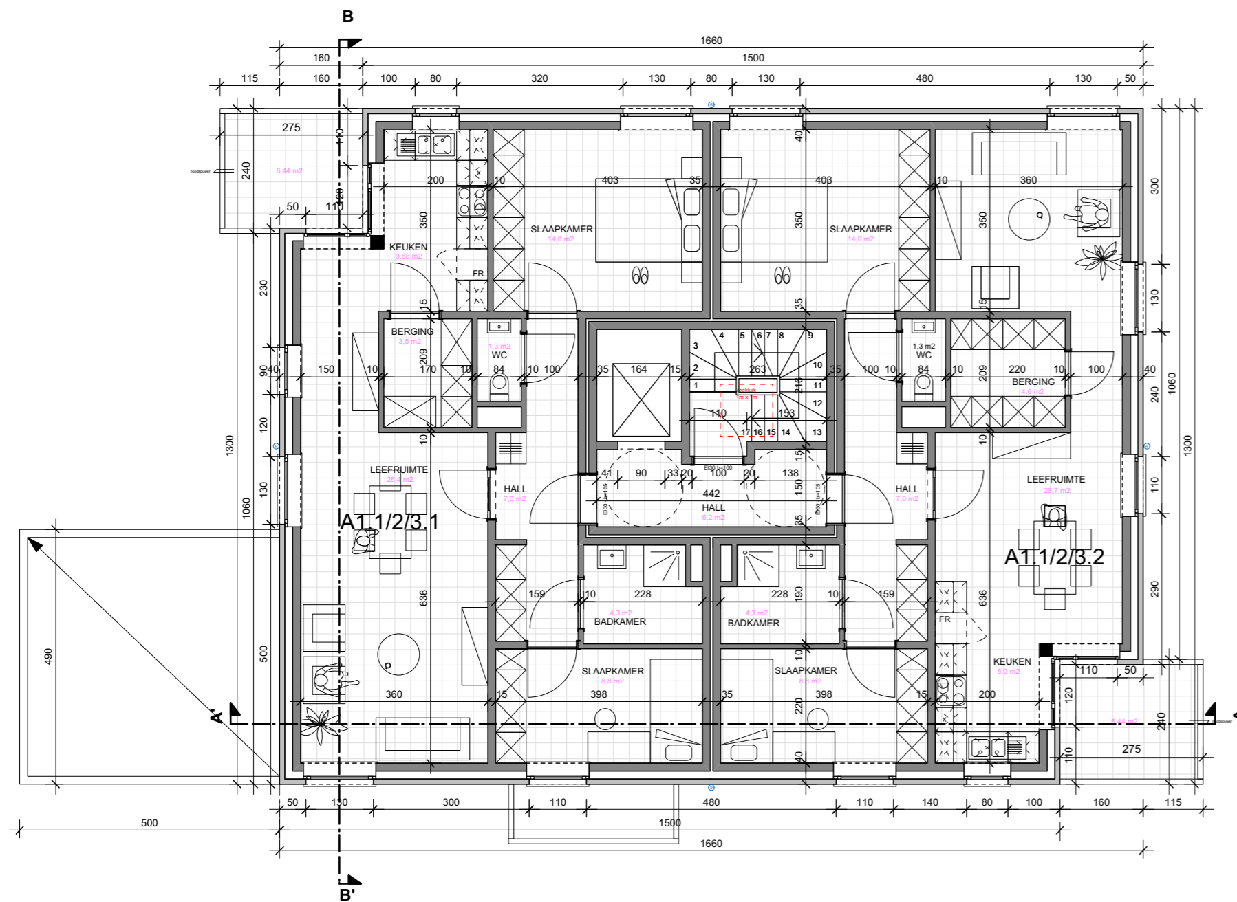
Appartementen Type A1 - VERDIEPING 1-3
