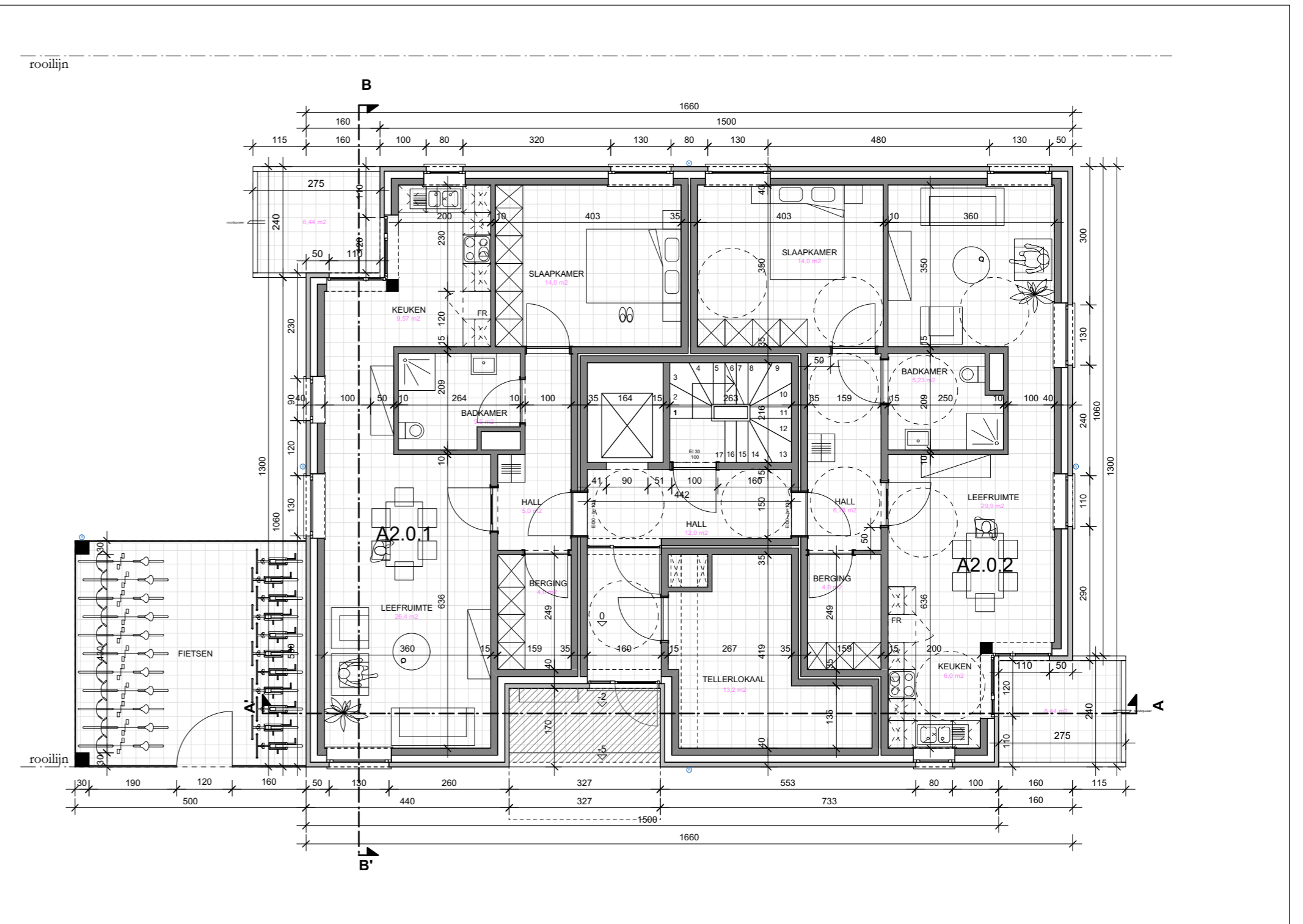
Appartementen Type A2 - GELIJKVLOERS (deels aangepast voor mindervaliden)
