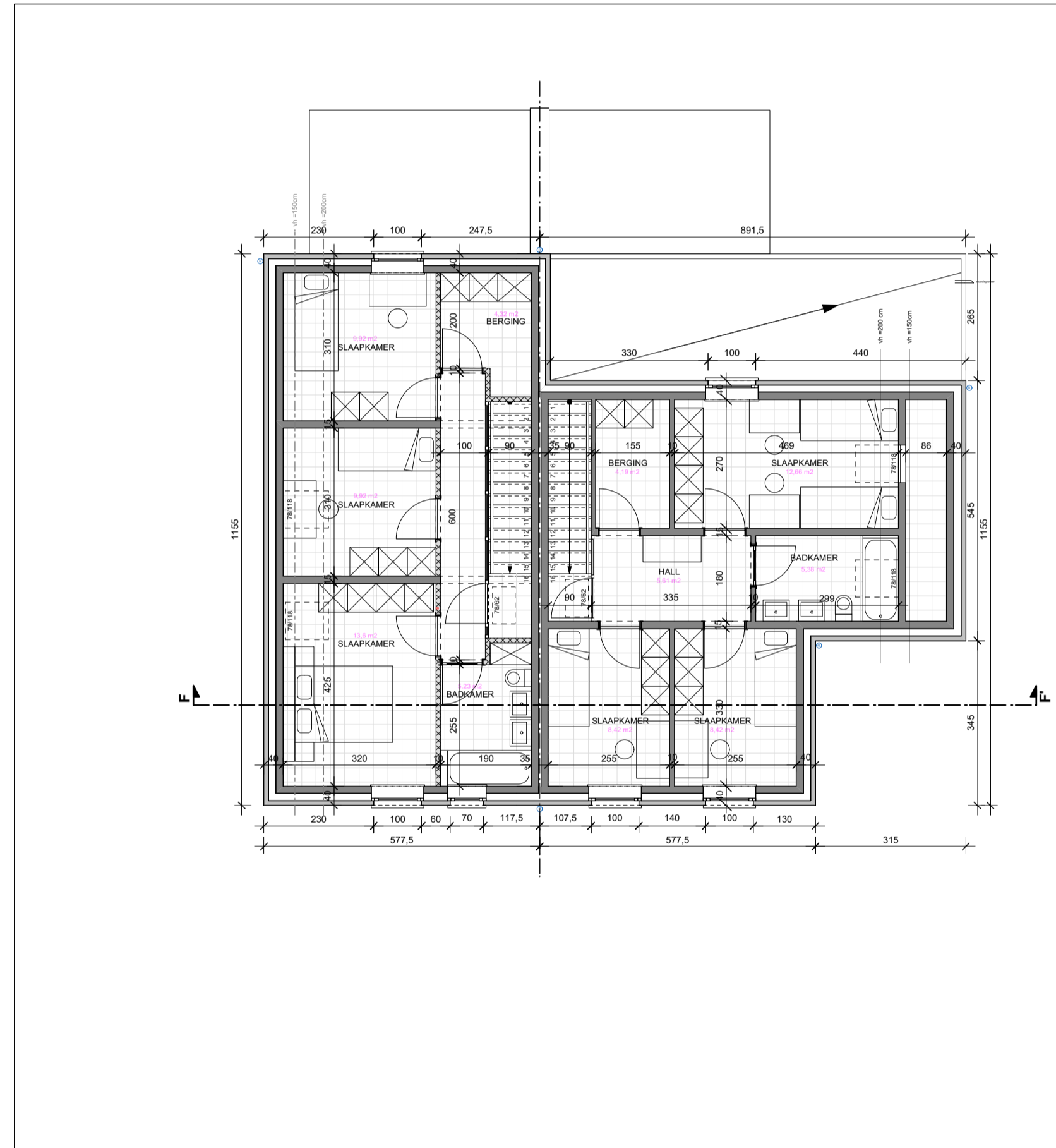
Typechakeling CD - VERDIEPING 1
