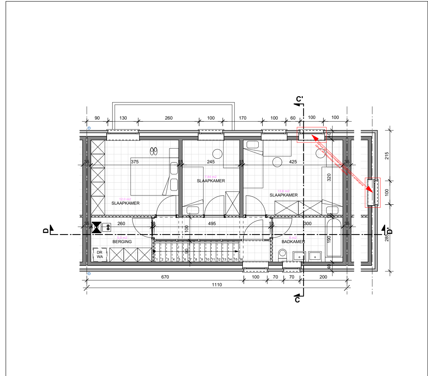
Rijwoningen Type B - VERDIEPING 1
