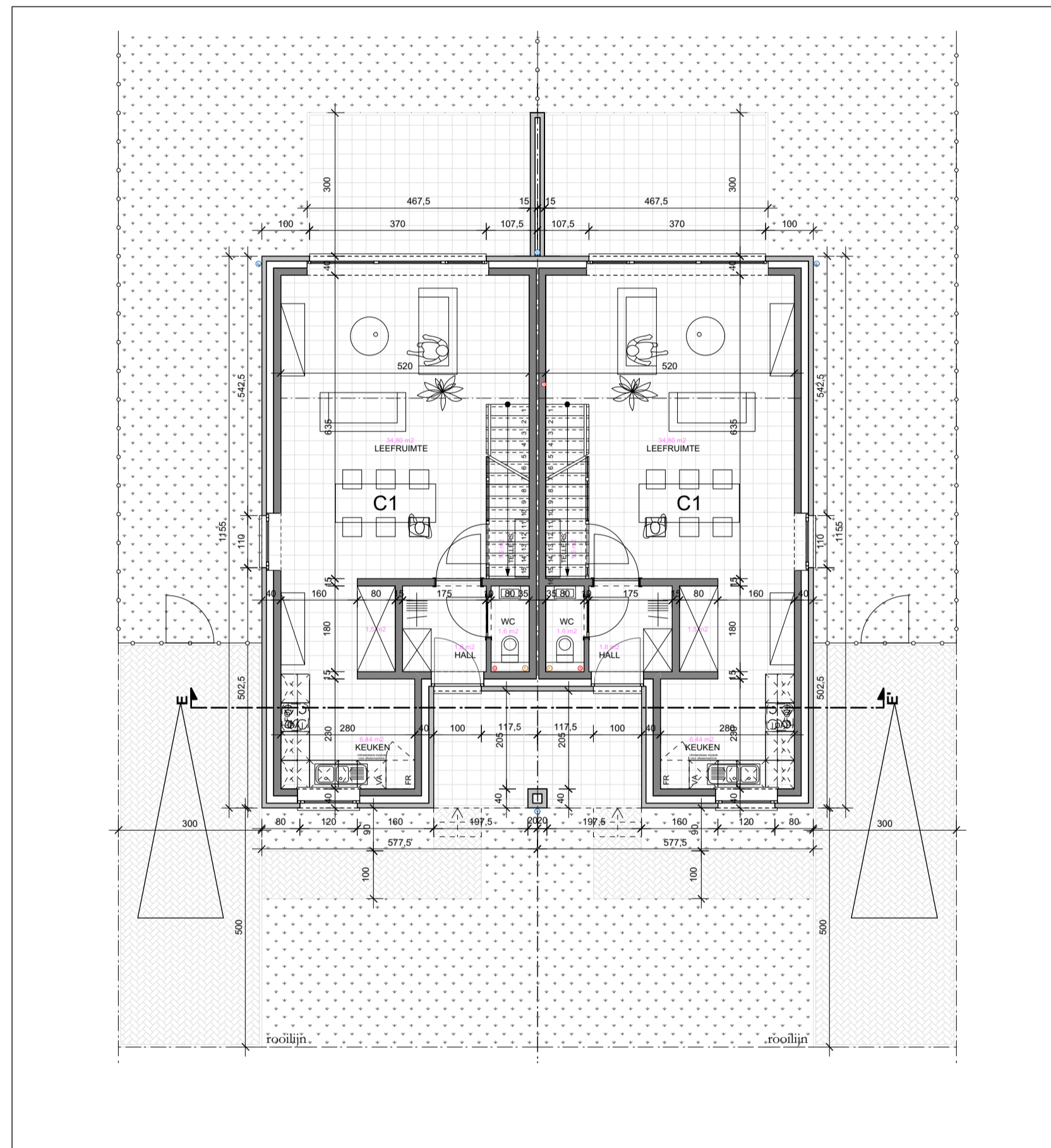
Typeschakeling CC - GELIJKVLOERS
