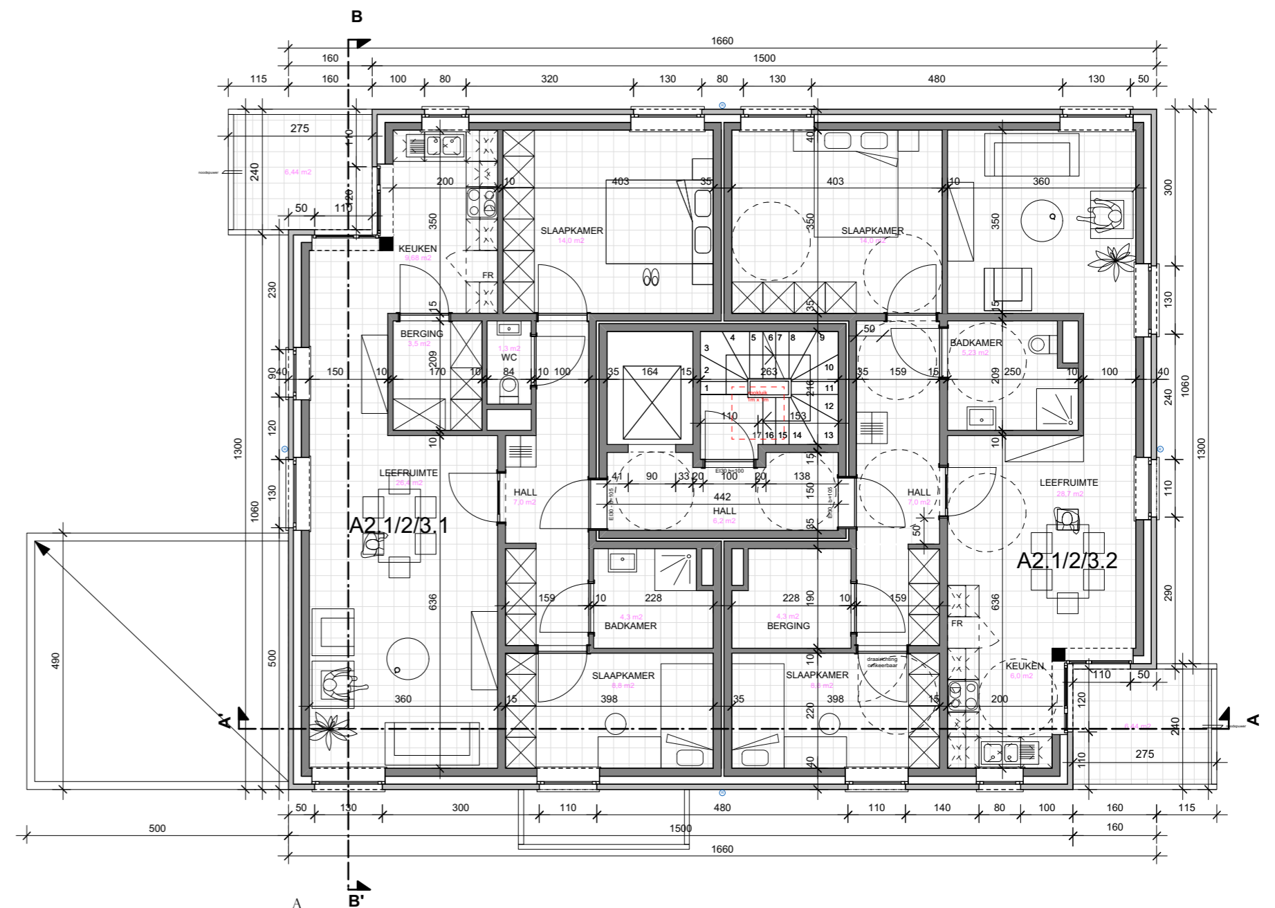
Appartementen Type A2 - VERDIEPING 1-3 (deels aangepast voor mindervaliden)
