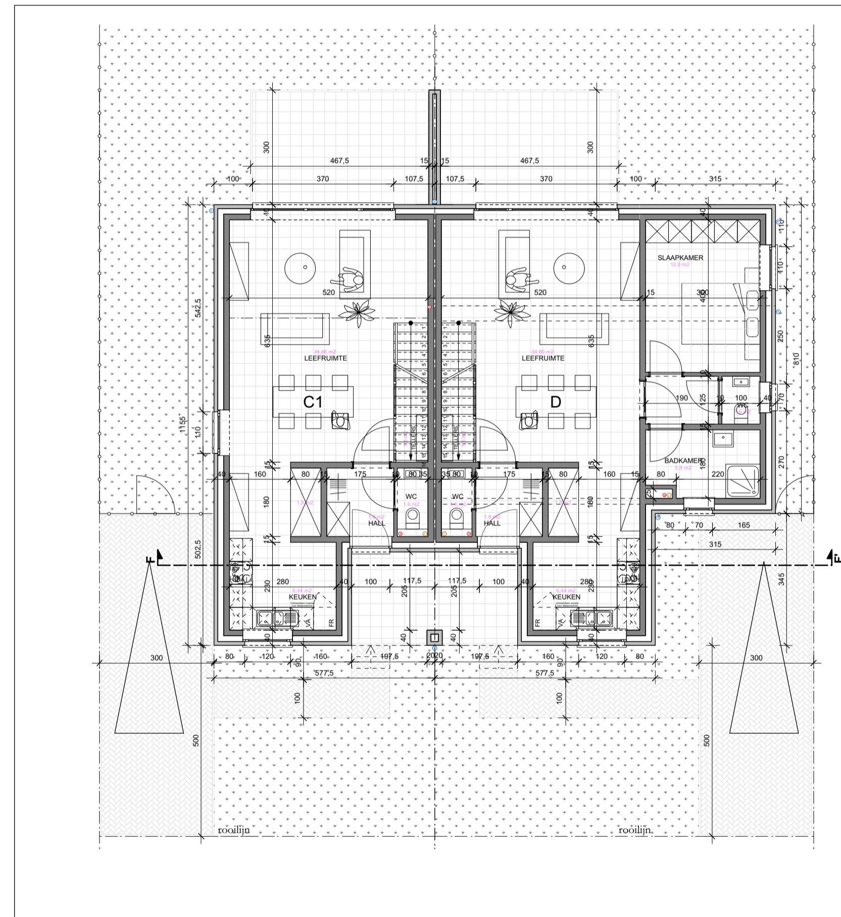
Typeschakeling CD - GELIJKVLOERS
