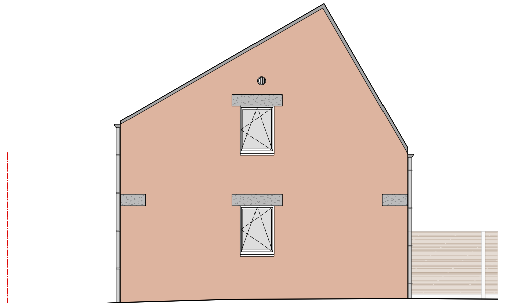
RECHTER-ZIJGEVEL (type G)
