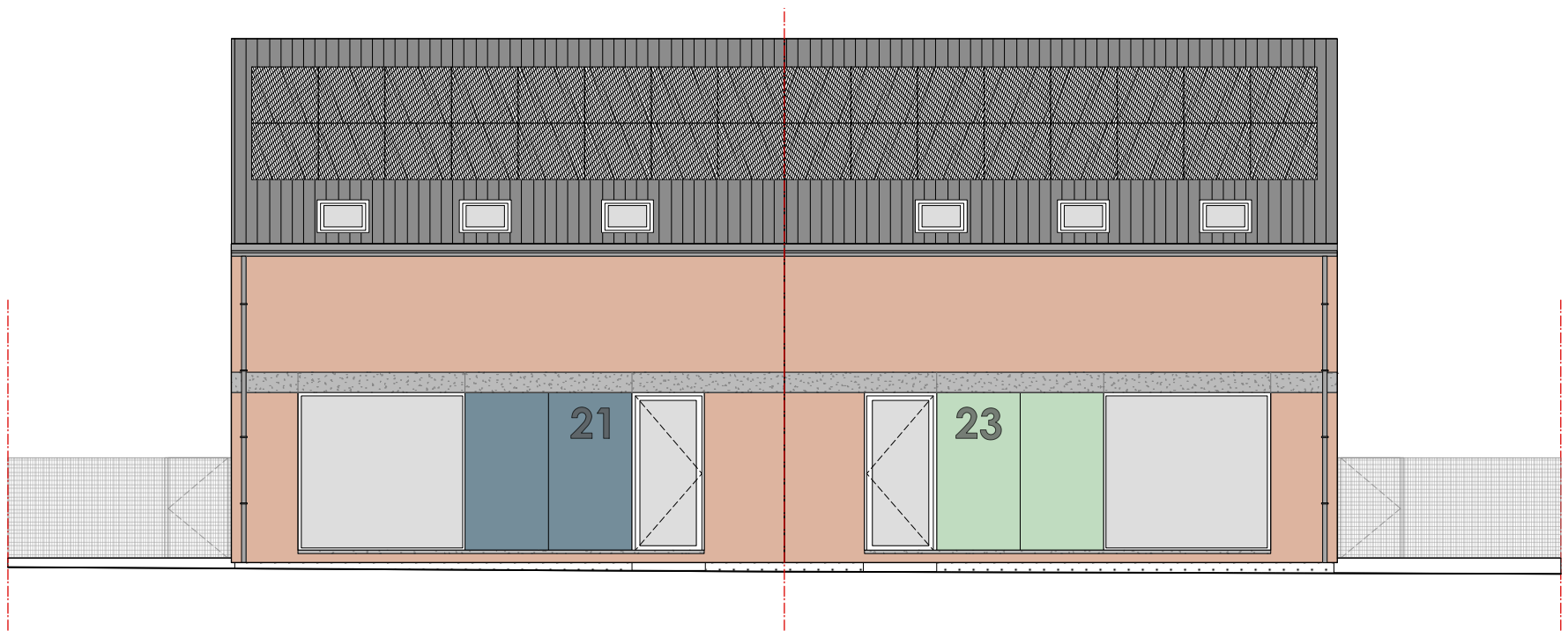
VOORGEVEL (type G)
