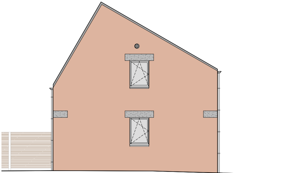
LINKER-ZIJGEVEL (type G)
